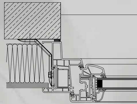
Schéma de pose sur neuf
