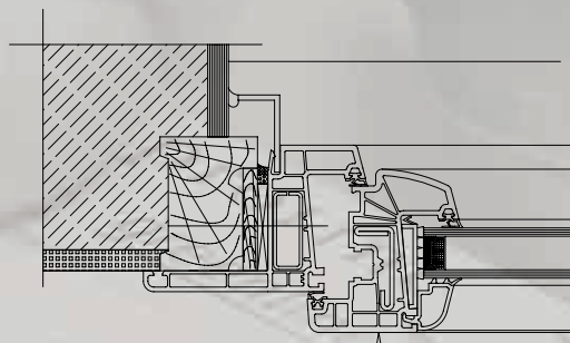
Schéma de pose en rénovation
